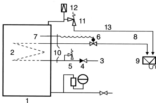
Abb. TA-Anschluss nass Ta-Anschluss drucklos möglich
