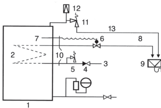
Abb. TA-Anschluss nass Ta-Anschluss drucklos möglich
